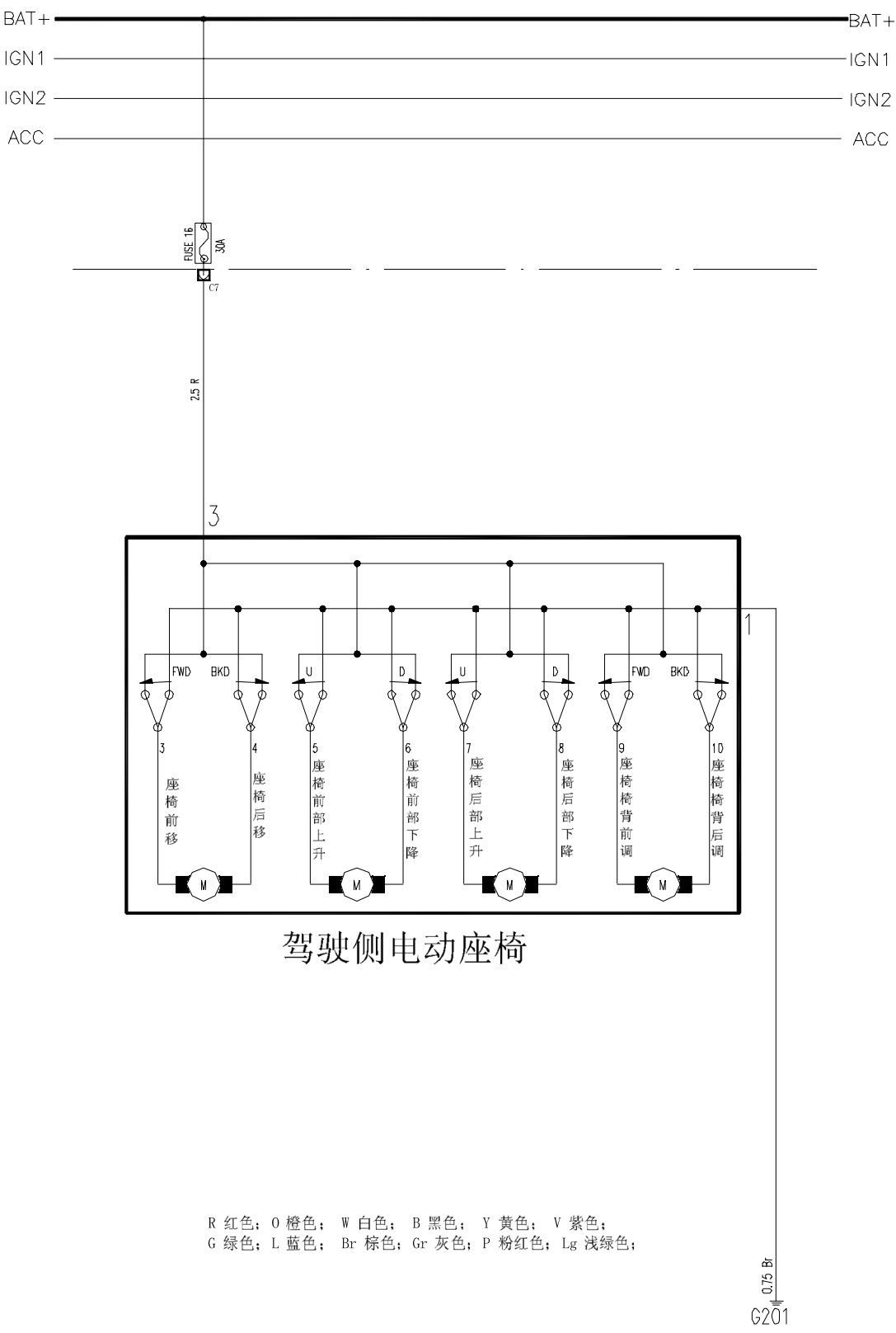
旗云5 1.8FC+MT 驾驶侧电动座椅 N0.03/09 电路图
